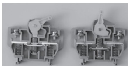
左：通電（オン）時 右：断路（オフ）時
