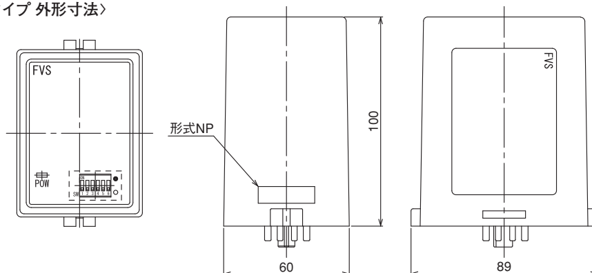
〈電圧設定 8ピンタイプ 外形寸法〉
