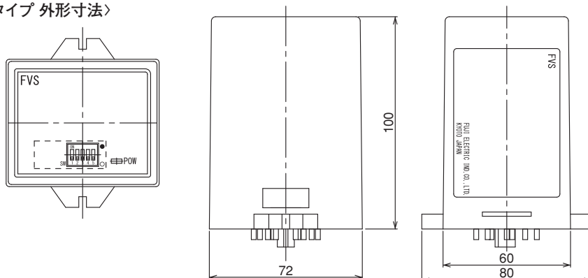
〈電圧設定 14ピンタイプ 外形寸法〉
