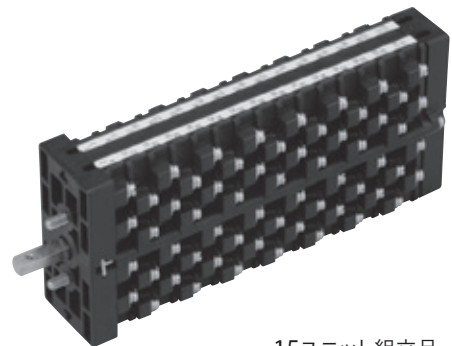
15ユニット組立品
