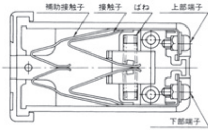
電流用接触端子図 (KTT-AW□)
