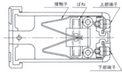
電圧用接触端子図 (KTT-VS□)
