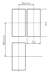
最小取付穴寸法 (単体取付時)
