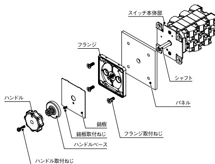
〈スイッチの取付方法〉
