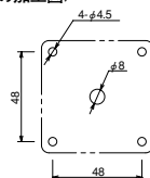
〈取付穴の加工図〉
