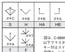
スイッチの施錠ポジション
