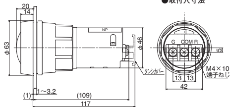
●取付寸寸法
