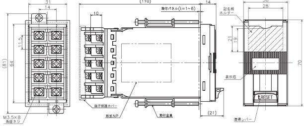
最小取付寸法 (単体取付時)
