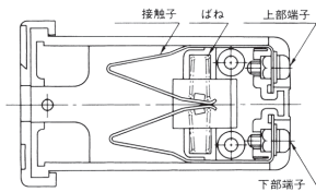
電圧用接触端子図 (KTT-VS□)
