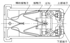
電流用接触端子図 (KTT-AW□)
