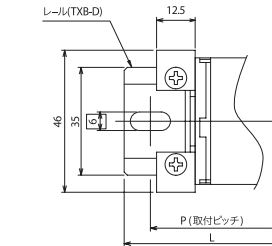
●組立寸法(代表寸法)
