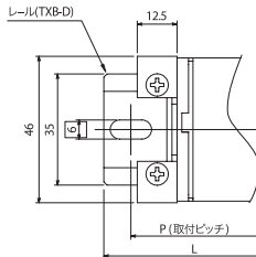
●組立寸法(代表寸法)
