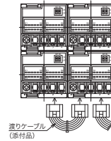
■裏面端子部
