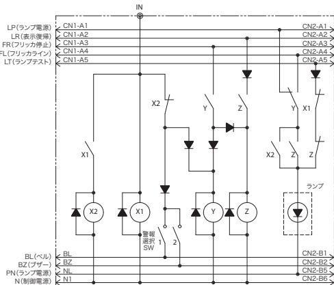
■回路図
