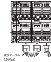
■裏面端子部
