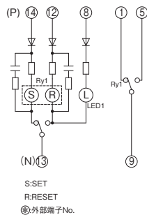
【1c接点仕様】
