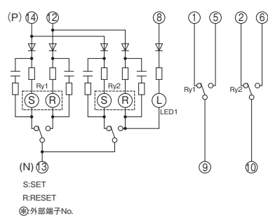
【2c接点仕様】
