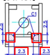
(組立側面視) リブ
