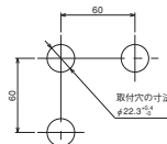
●取付パネル孔 (最小取付ピッチ)
