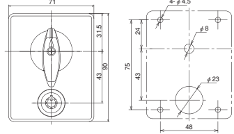
取付穴寸法
