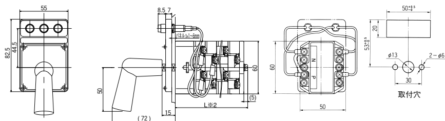
24V仕様
