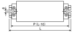
組立品Uカットレール TXB-F による組立
