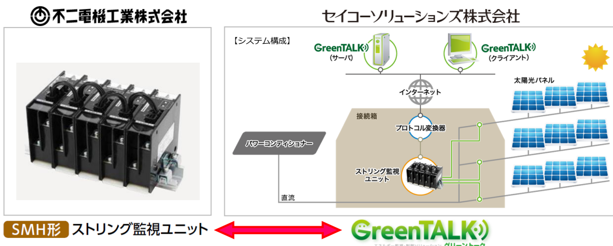
図：String監視ユニット「SMH形」と「GreenTALK」の接続イメージ
