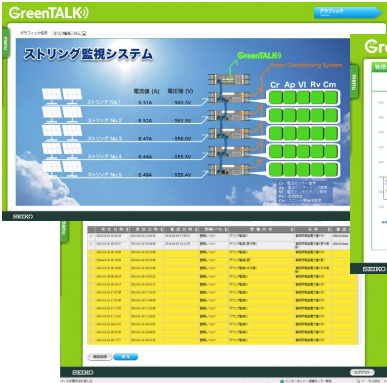
【 スtring監視モニタ 】
