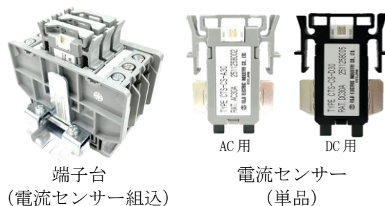
【電流計測端子台 CTS形】
